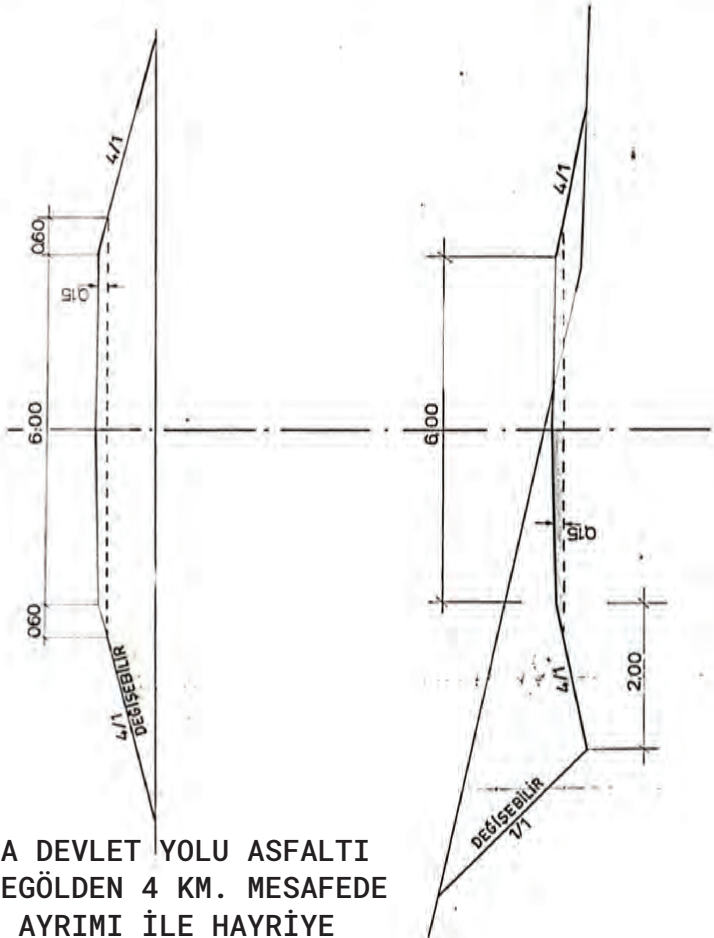
YENİ YAPILACAK YOLA TATBİK EDİLECEK EN KESİT TİPLERİ
